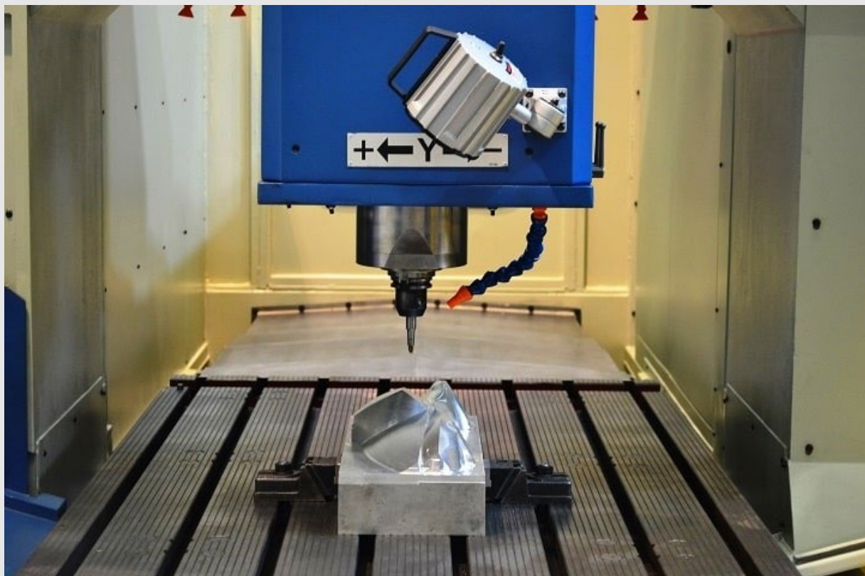
Ejemplo de fresadora de alta velocidad CORREA EURO2000 tras su reconstrucción
