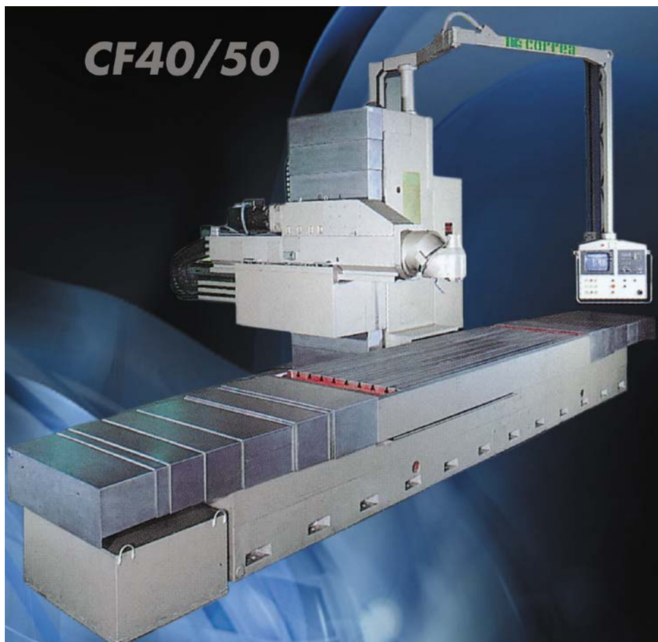
Fresadora CORREA CF40/50
