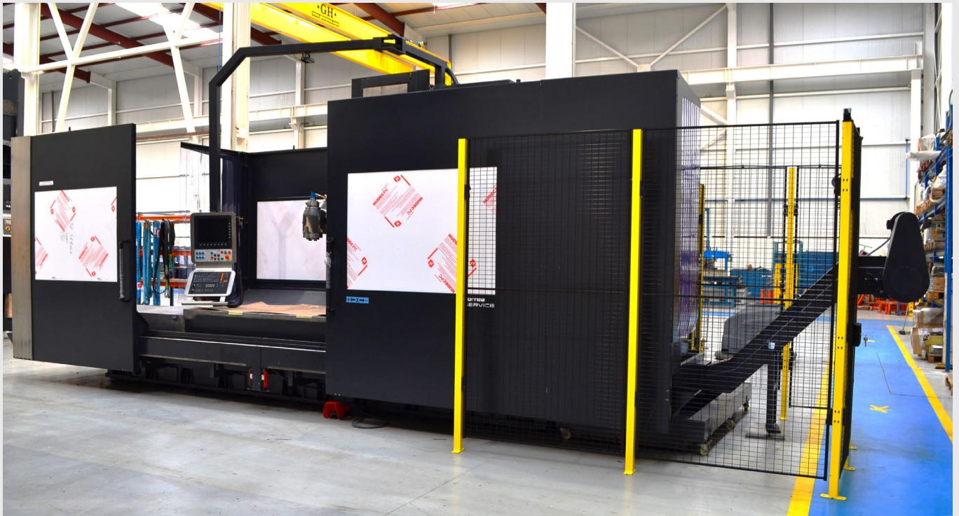
Reconstrucción de fresadora CORREA CF25/25 con cabezal manual (U22)
