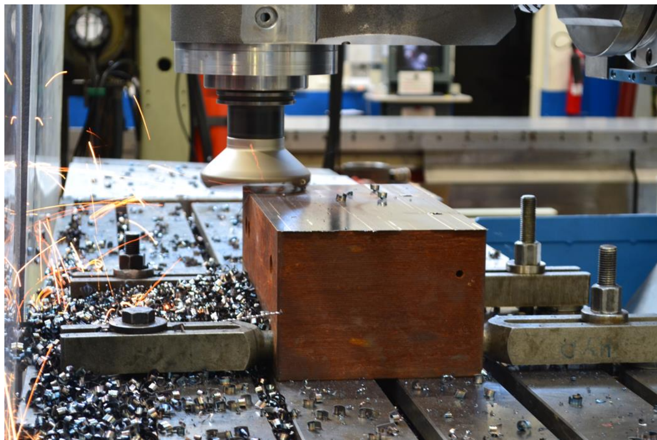
Fresadora CORREA CF 22/25-Plus
