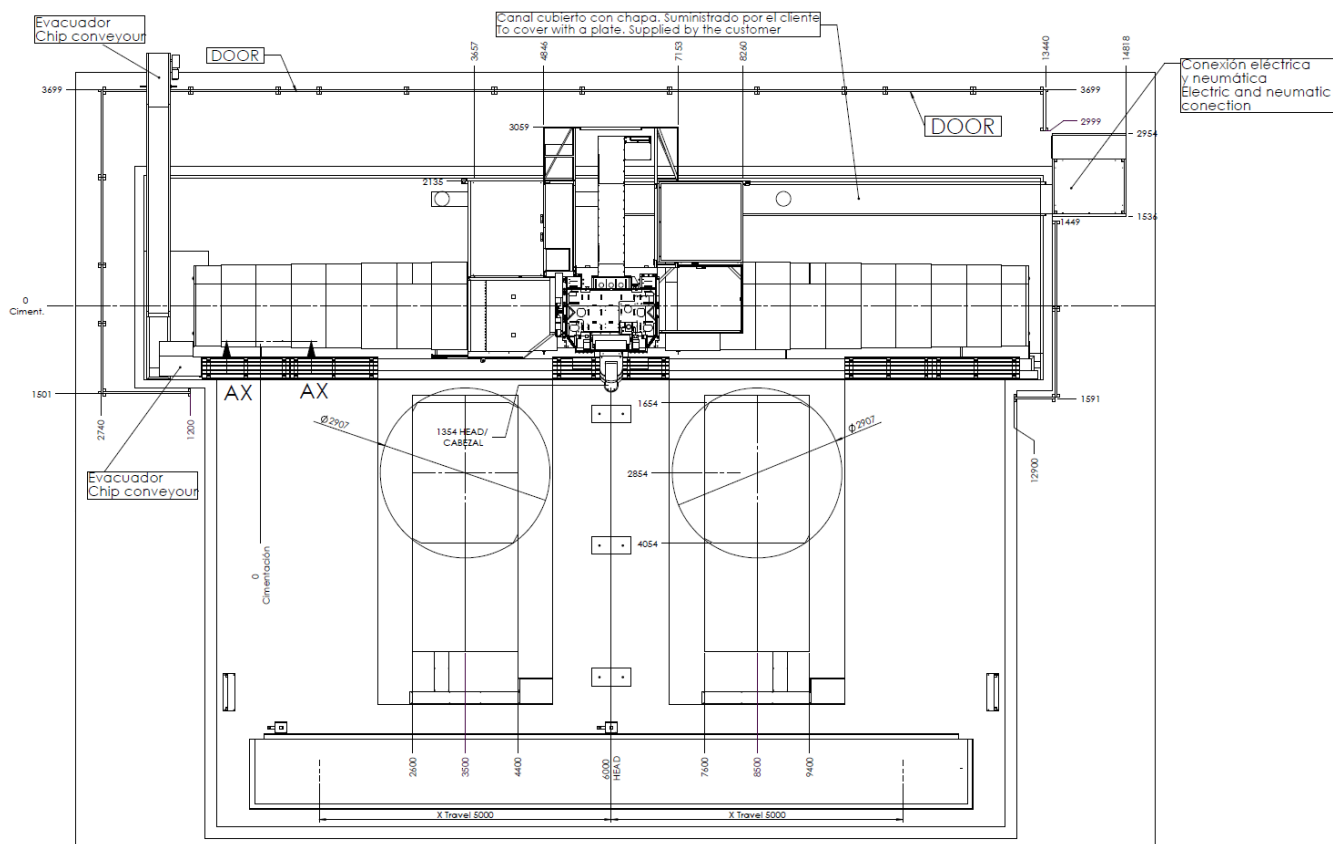
Fresadora CORREA AXIA 100 - Layout
