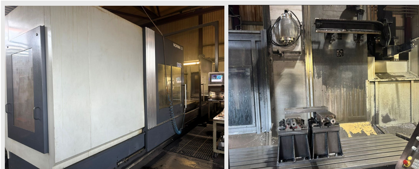
Esta fresadora CORREA NORMA35 en origen, antes de su reconstrucción
